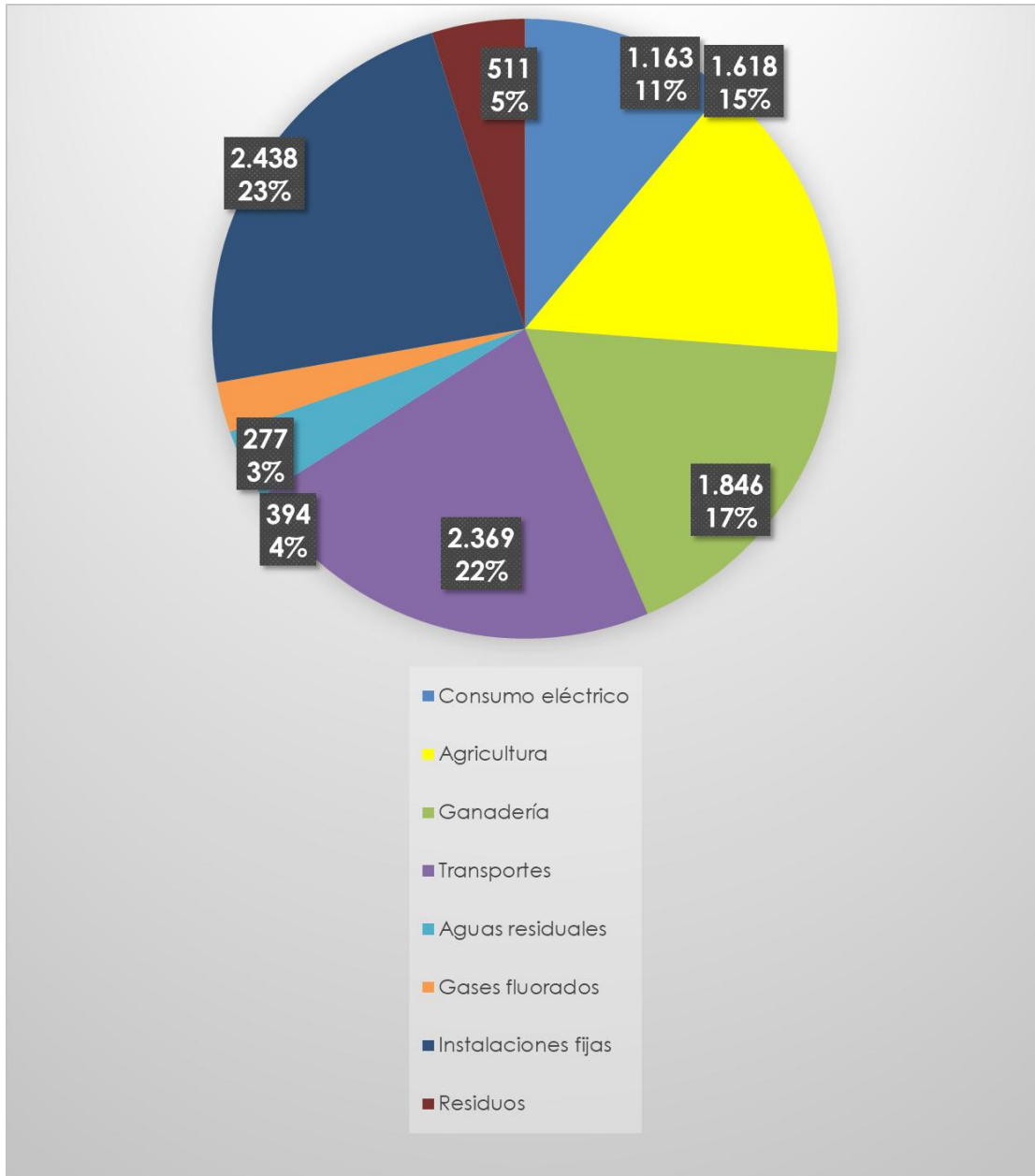
Figura 5. Huella de carbono. Fuente: CMA. Elaboración propia.
