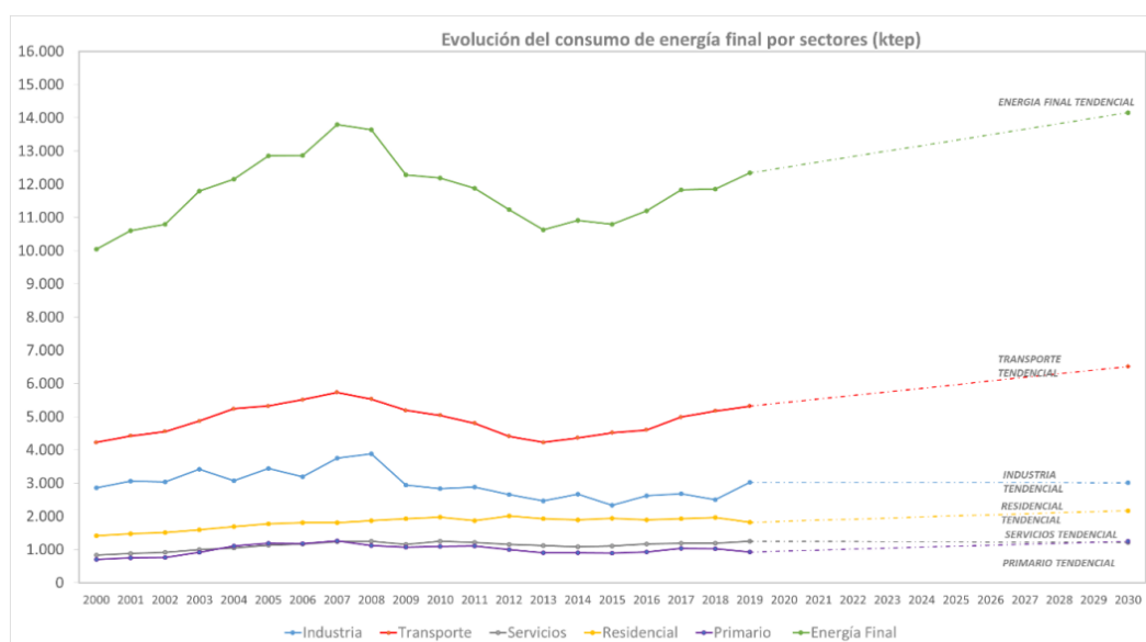
Figura 6. Evolución del consumo final por sectores. Fuente. Guía PMCC.
