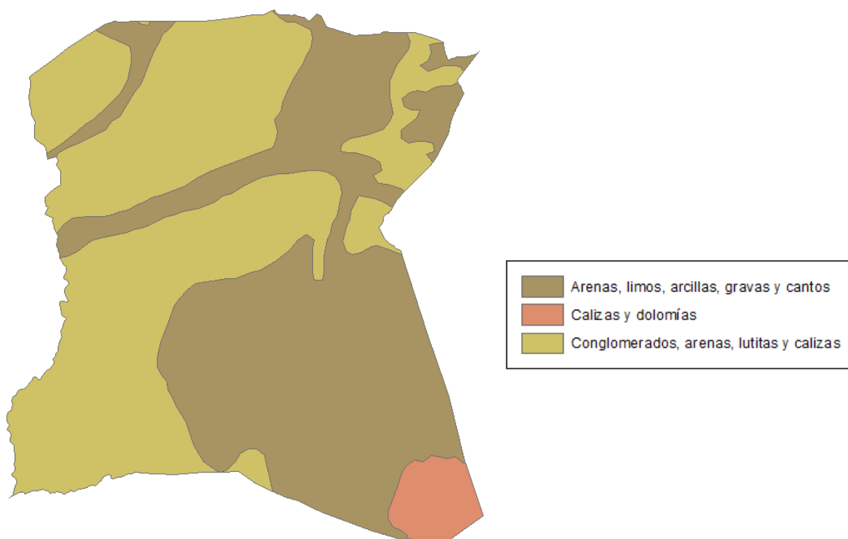
Mapa 1. Geología del municipio de Galera.
